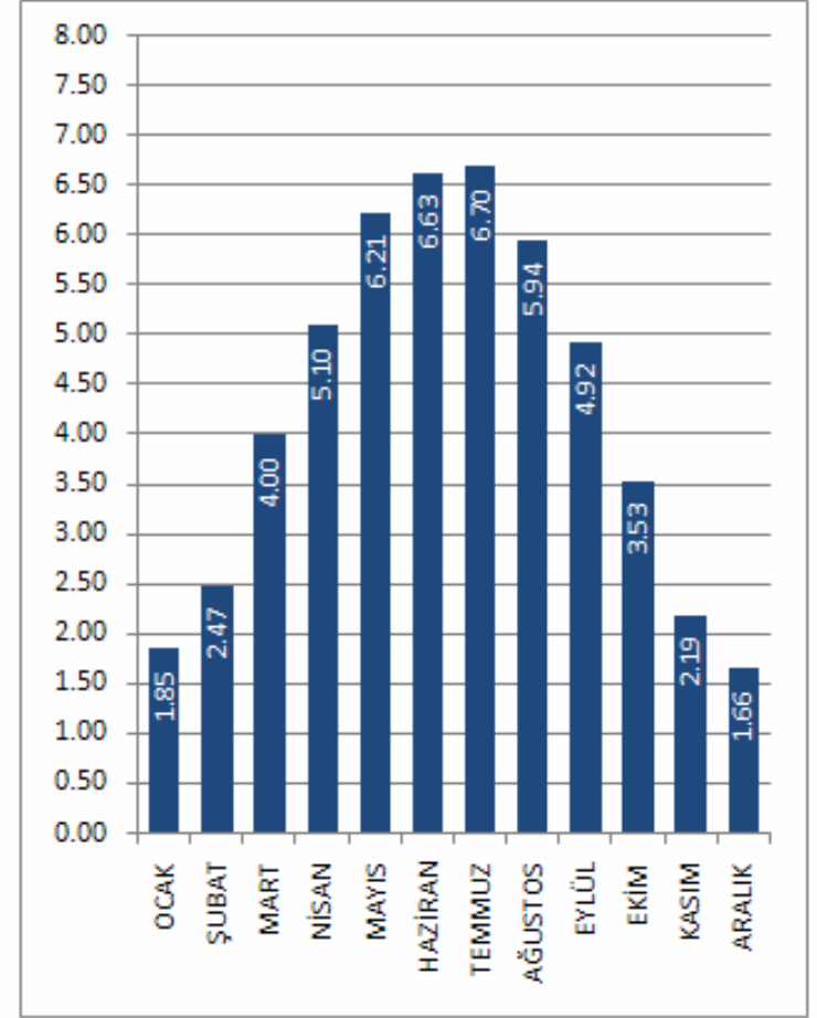
AFYON İLİ GLOBAL RADYASYON DEĞERLERİ (KWh/m 2 -gün)
