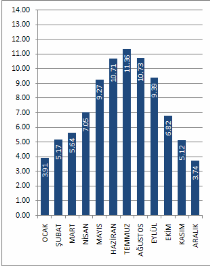
AFYON İLİ GÜNEŞLENME SÜRESİ DEĞERLERİ (Saat)
