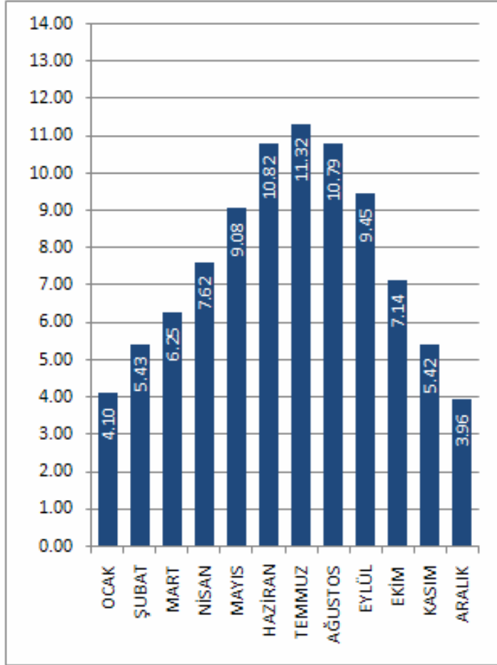
AĞRI İLİ GÜNEŞLENME SÜRESİ DEĞERLERİ (Saat)
