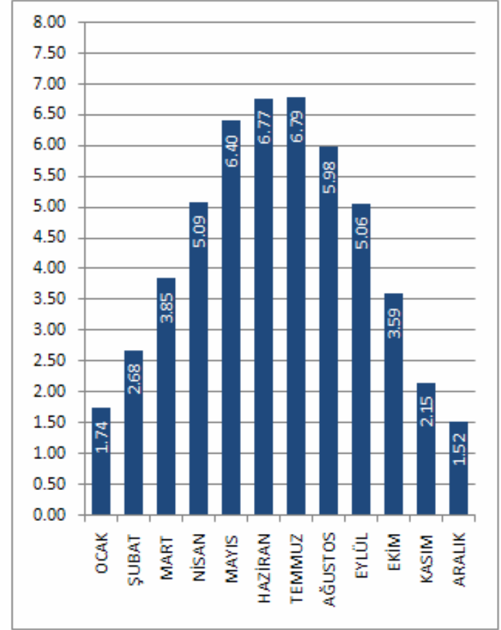
AĞRI İLİ GLOBAL RADYASYON DEĞERLERİ (KWh/m 2 -gün)
