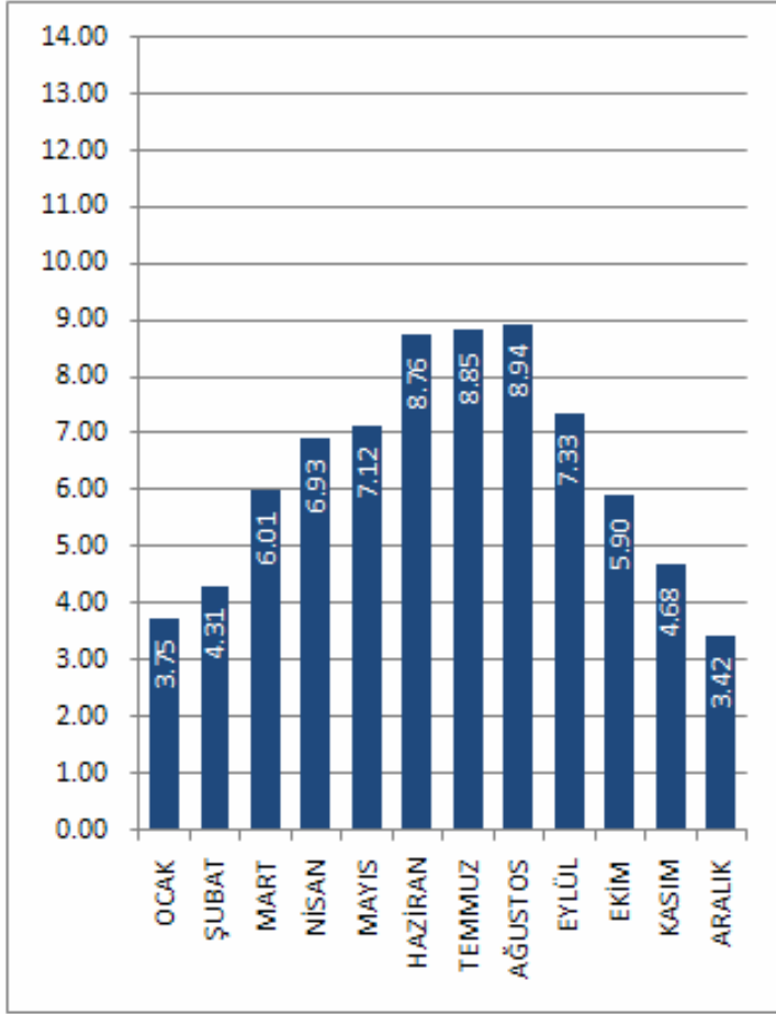
ARDAHAN İLİ GÜNEŞLENME SÜRESİ DEĞERLERİ (Saat)
