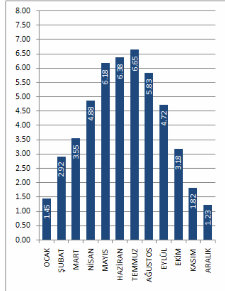
ARDAHAN İLİ GLOBAL RADYASYON DEĞERLERİ (KWh/m 2 -gün)
