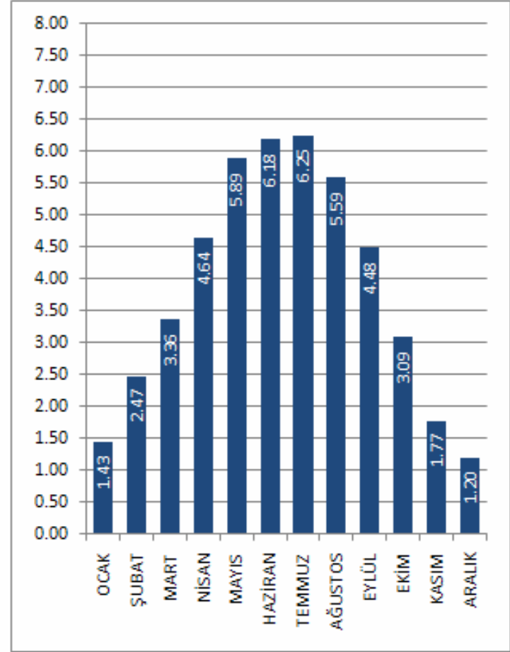
ARTVİN İLİ GLOBAL RADYASYON DEĞERLERİ (KWh/m 2 -gün)
