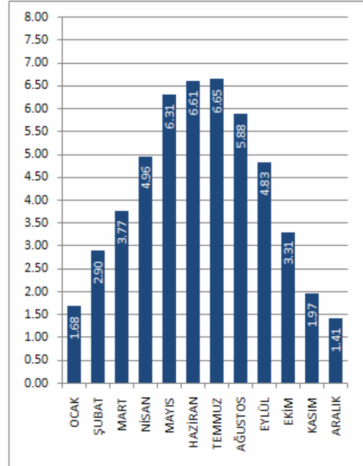
BAYBURT İLİ GLOBAL RADYASYON DEĞERLERİ (KWh/m 2 -gün)
