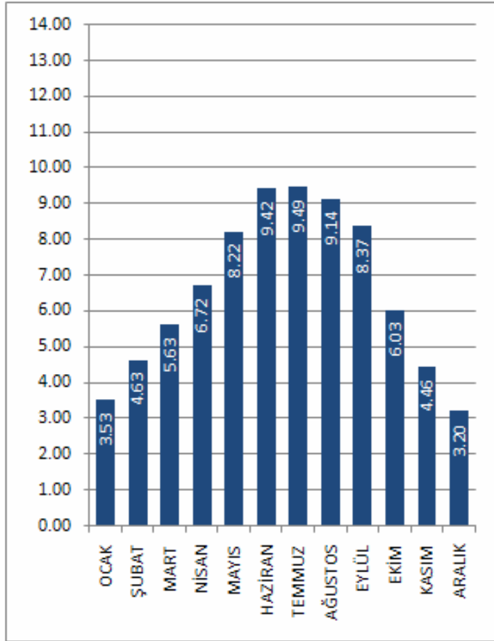
BAYBURT İLİ GÜNEŞLENME SÜRESİ DEĞERLERİ (Saat)
