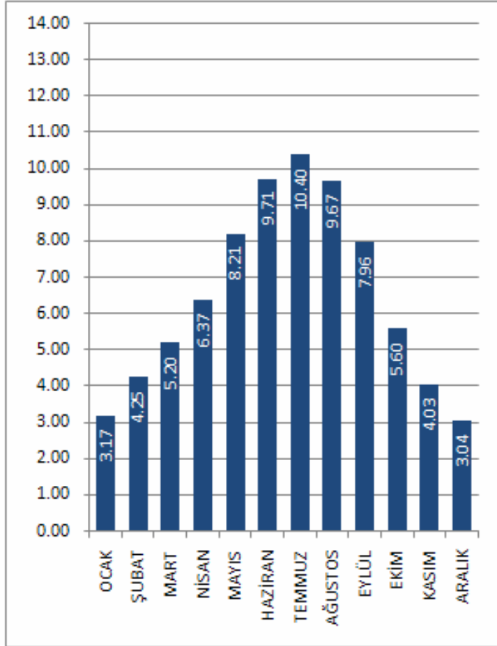
DÜZCE İLİ GÜNEŞLENME SÜRESİ DEĞERLERİ (Saat)
