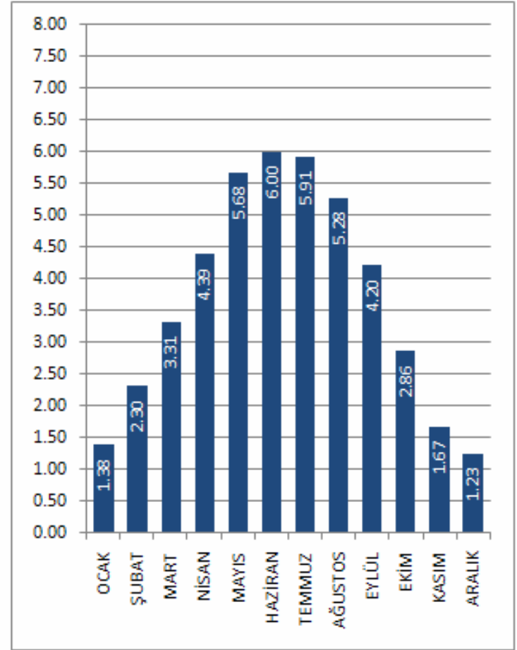
DÜZCE İLİ GLOBAL RADYASYON DEĞERLERİ (KWh/m 2 -gün)
