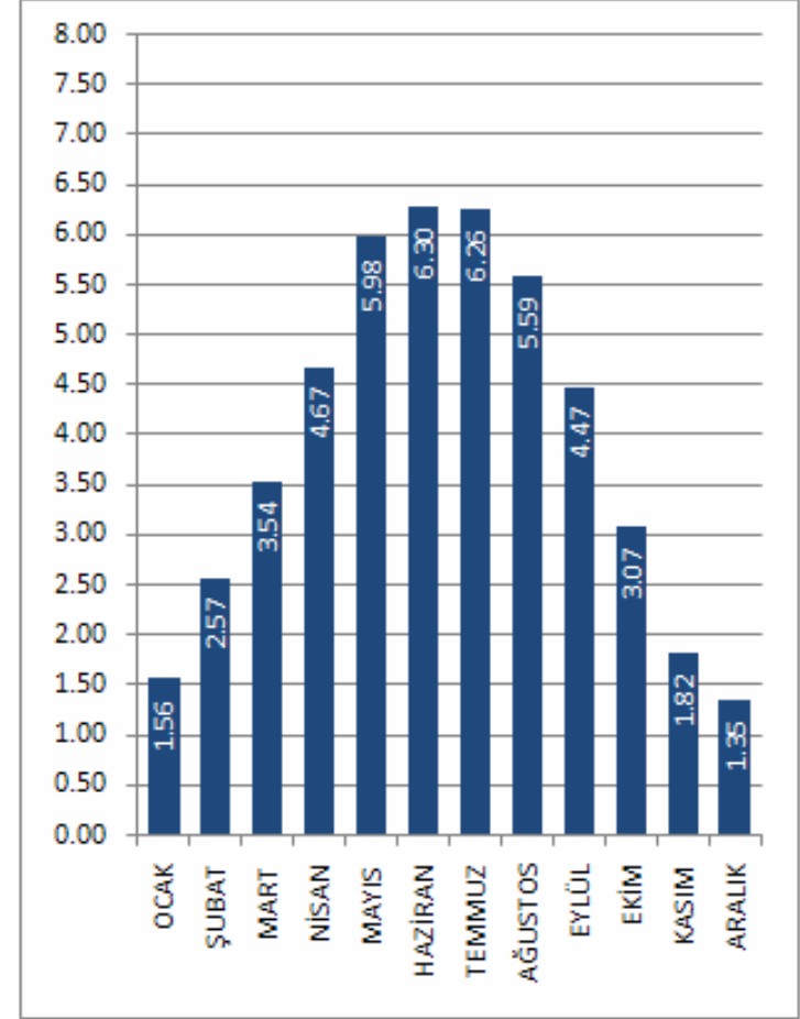
GİRESUN İLİ GLOBAL RADYASYON DEĞERLERİ (KWh/m 2 -gün)
