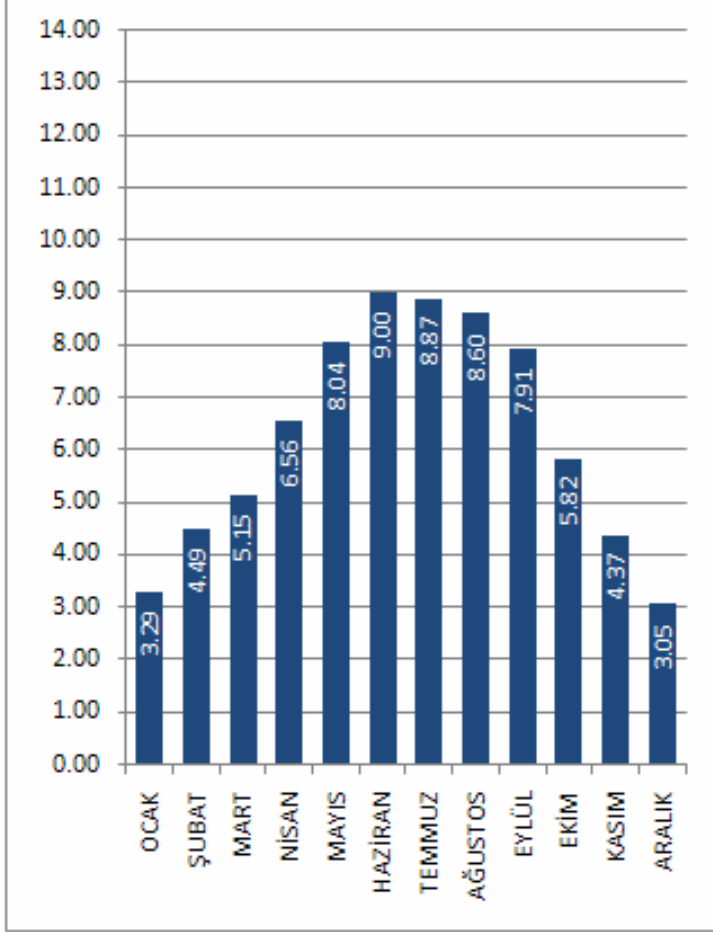
GİRESUN İLİ GÜNEŞLENME SÜRESİ DEĞERLERİ (Saat)
