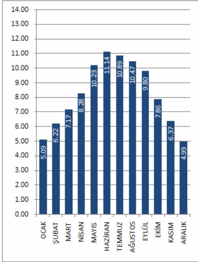
HATAY İLİ GÜNEŞLENME SÜRESİ DEĞERLERİ (Saat)
