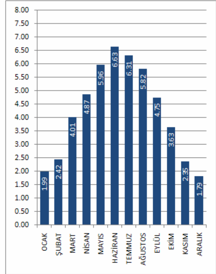
HATAY İLİ GLOBAL RADYASYON DEĞERLERİ (KWh/m 2 -gün)
