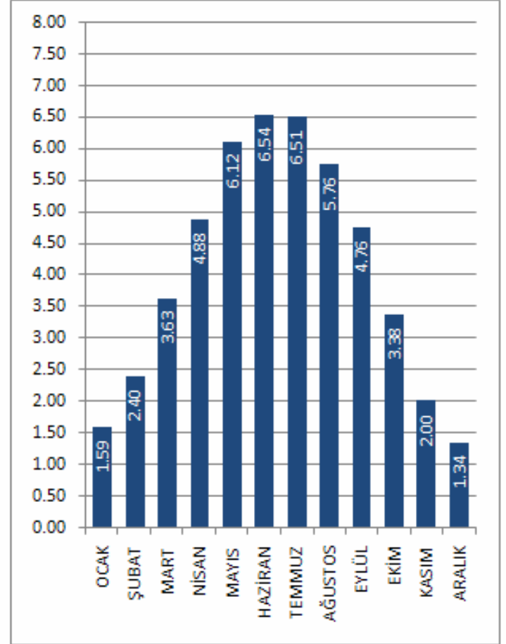
İĞDIR İLİ GLOBAL RADYASYON DEĞERLERİ (KWh/m 2 -gün)
