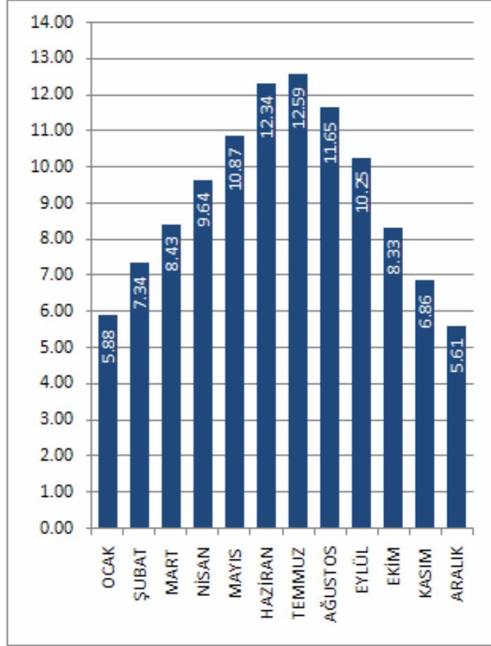
İĞDIR İLİ GÜNEŞLENME SÜRESİ DEĞERLERİ (Saat)
