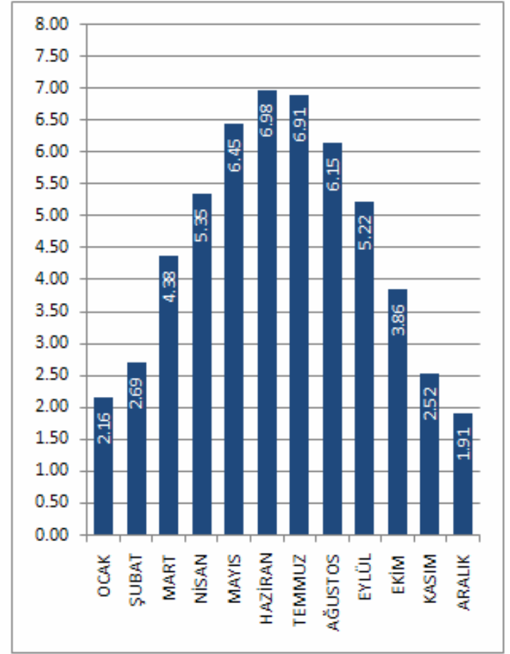
KARAMAN İLİ GLOBAL RADYASYON DEĞERLERİ (KWh/m 2 -gün)
