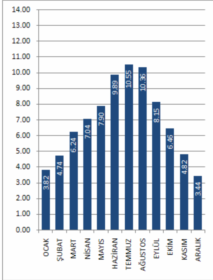
KARS İLİ GÜNEŞLENME SÜRESİ DEĞERLERİ (Saat)
