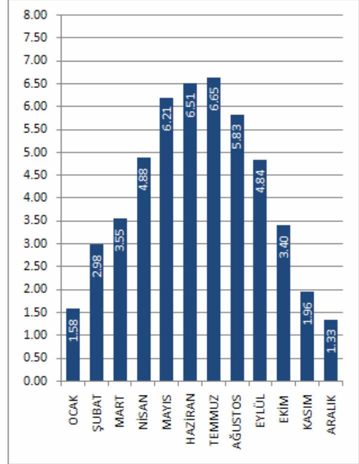
KARS İLİ GLOBAL RADYASYON DEĞERLERİ (KWh/m 2 -gün)
