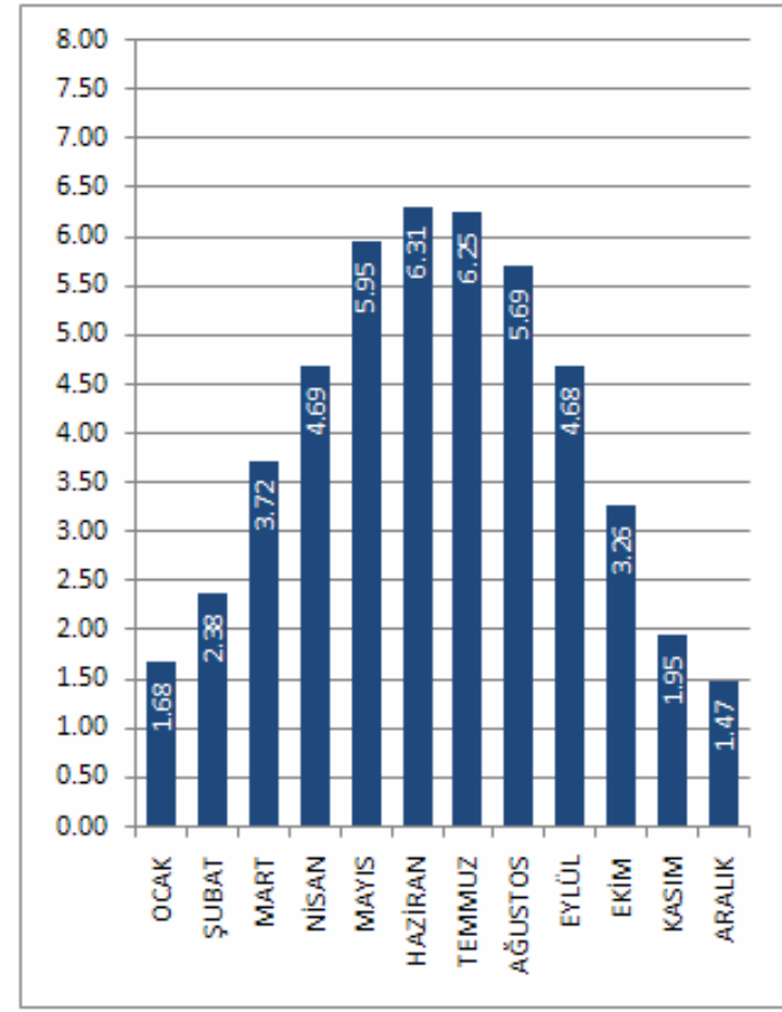
KIRIKKALE İLİ GLOBAL RADYASYON DEĞERLERİ (KWh/m 2 -gün)
