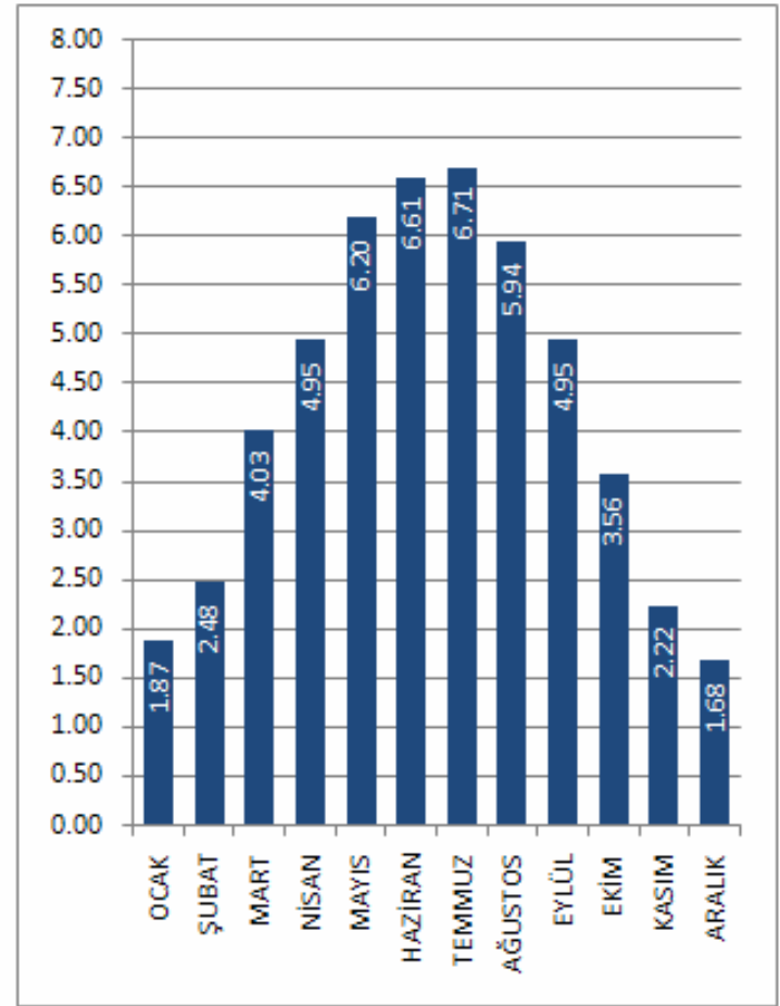
NEVŞEHİR İLİ GLOBAL RADYASYON DEĞERLERİ (KWh/m 2 -gün)
