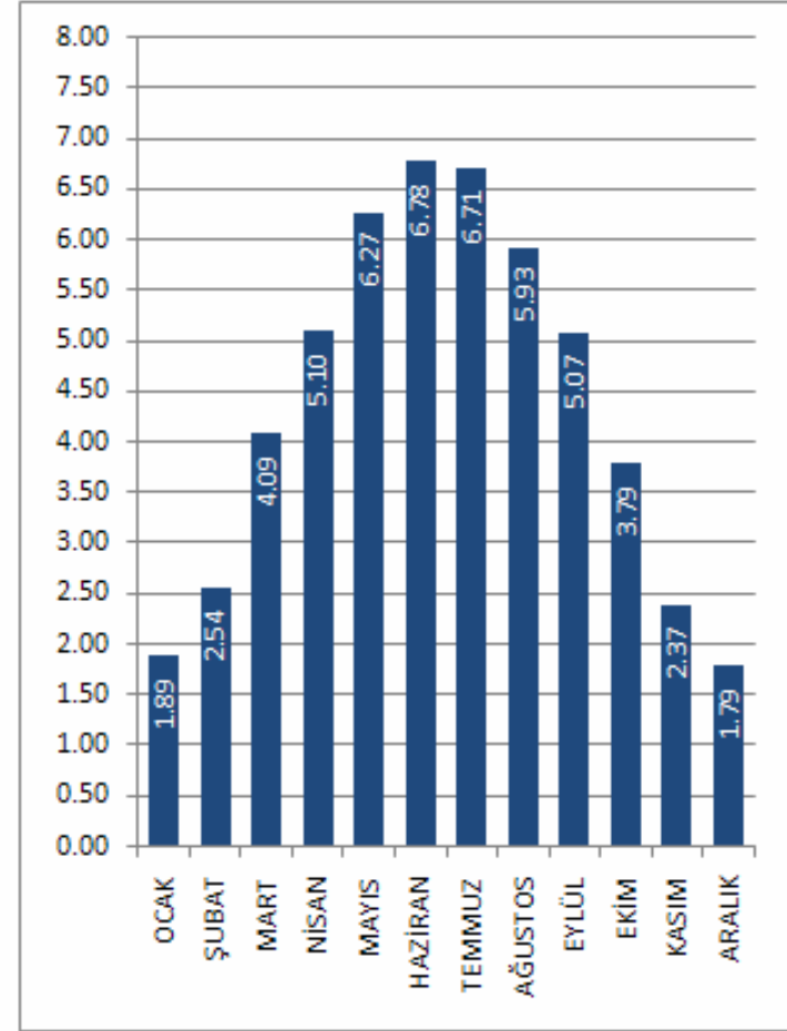
SIIRT İLİ GLOBAL RADYASYON DEĞERLERİ (KWh/m 2 -gün)
