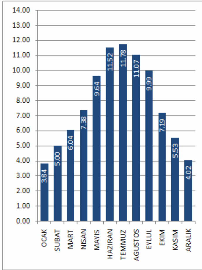
SIIRT İLİ GÜNEŞLENME SÜRESİ DEĞERLERİ (Saat)
