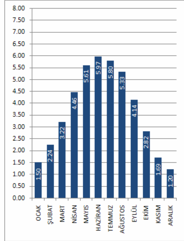
TEKİRDAĞ İLİ GLOBAL RADYASYON DEĞERLERİ (KWh/m 2 -gün)
