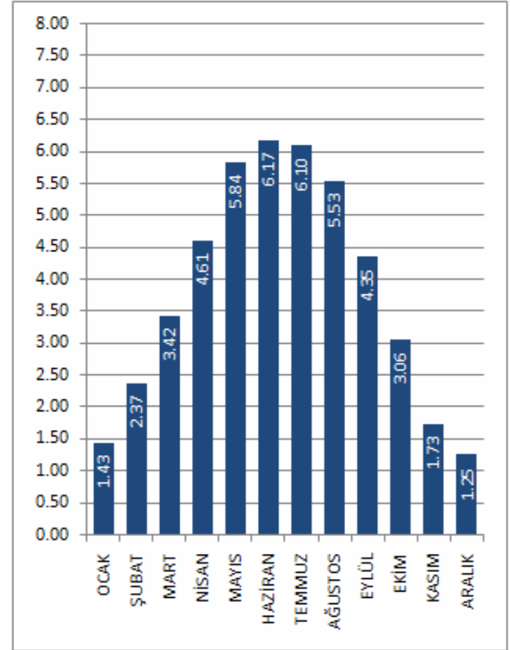
TRABZON İLİ GLOBAL RADYASYON DEĞERLERİ (KWh/m 2 -gün)
