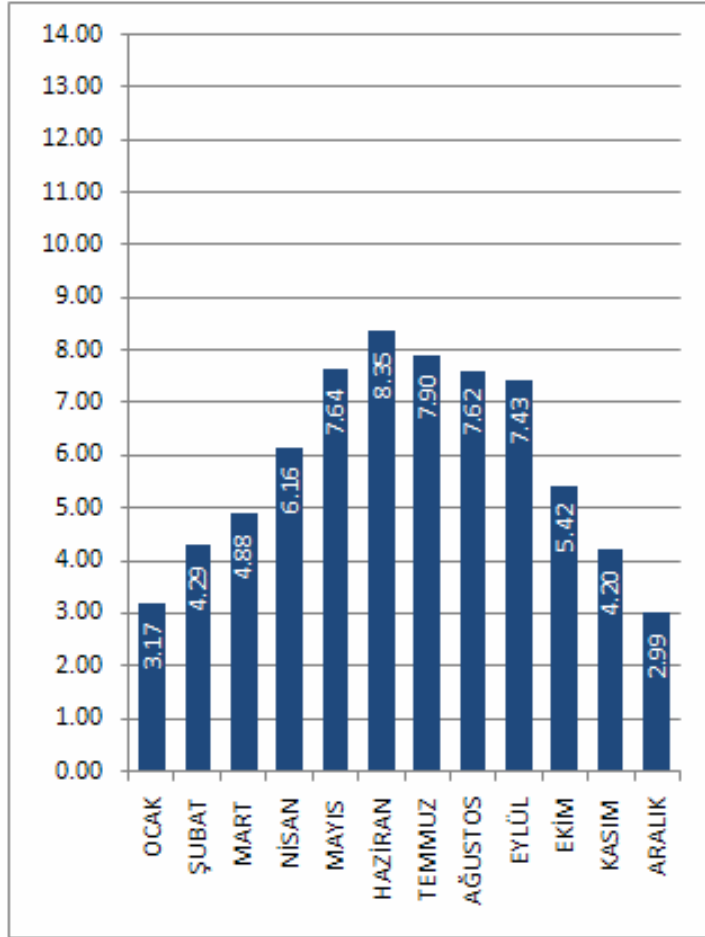
TRABZON İLİ GÜNEŞLENME SÜRESİ DEĞERLERİ (Saat)
