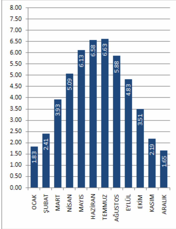
UŞAK İLİ GLOBAL RADYASYON DEĞERLERİ (KWh/m 2 -gün)
