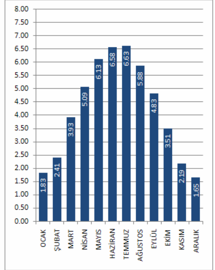
UŞAK İLİ GLOBAL RADYASYON DEĞERLERİ (KWh/m 2 -gün)
