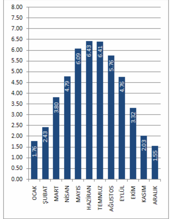
YOZGAT İLİ GLOBAL RADYASYON DEĞERLERİ (KWh/m 2 -gün)
